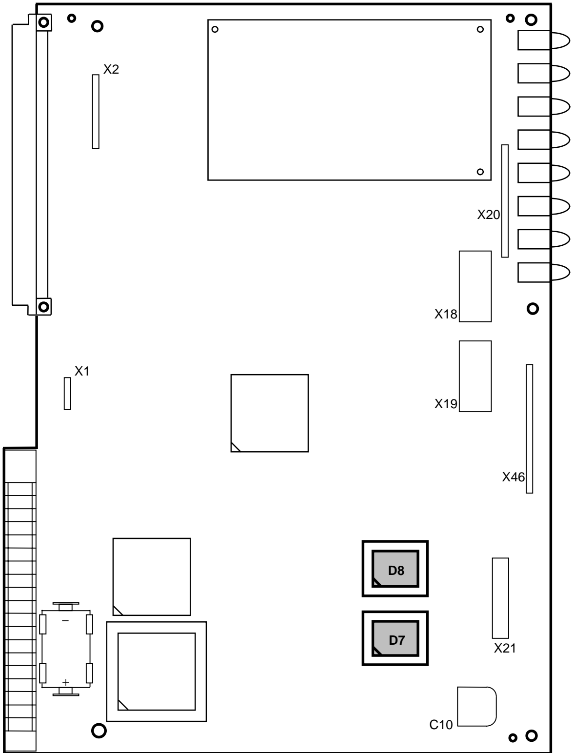
Bild 2: KSP2-Leiterplatte, Bauelementeseite und Lage der EPROMs D7 und D8
