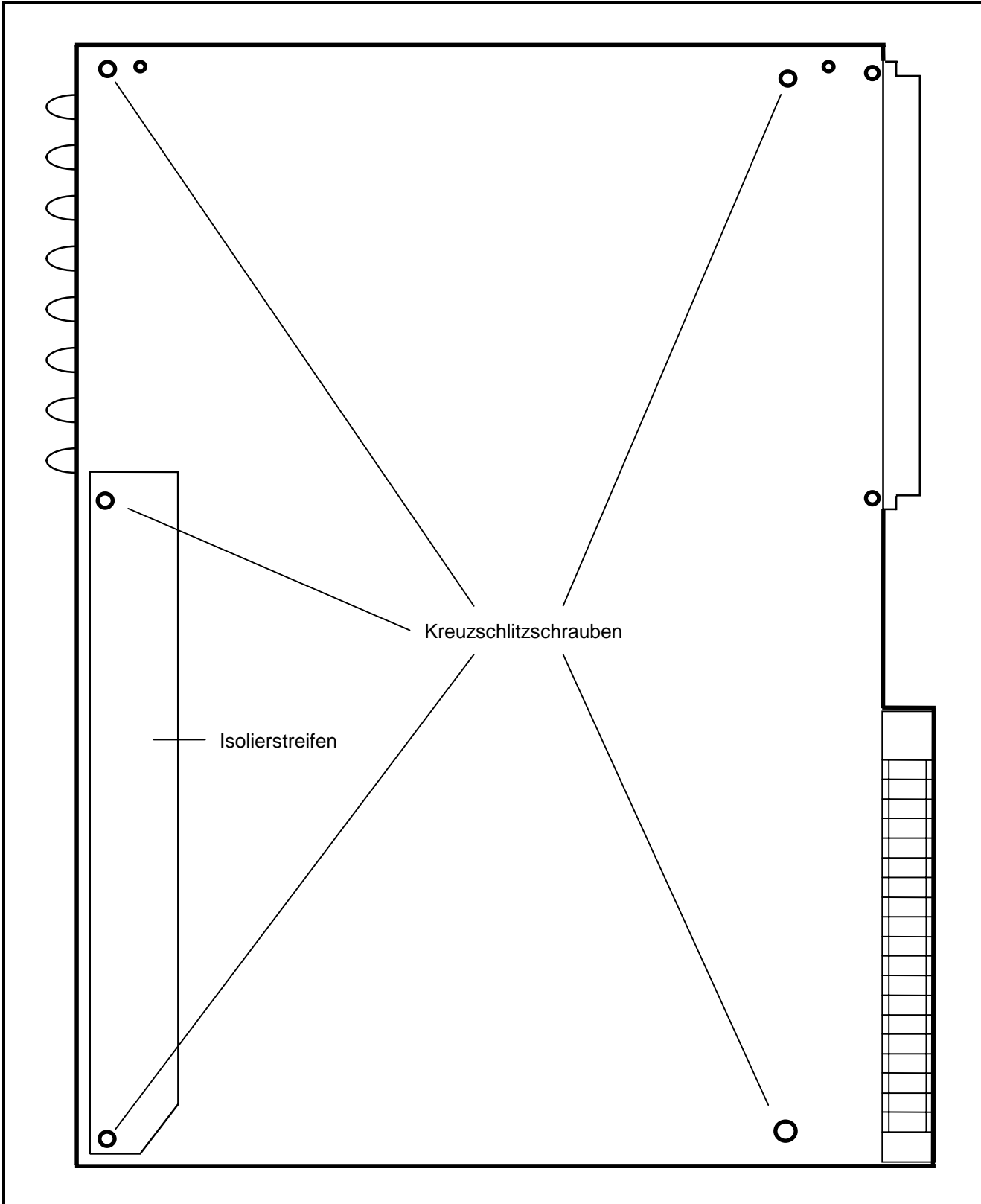
Bild1: KSP2-Leiterplatte, Rückseite mit Befestigungsschrauben
