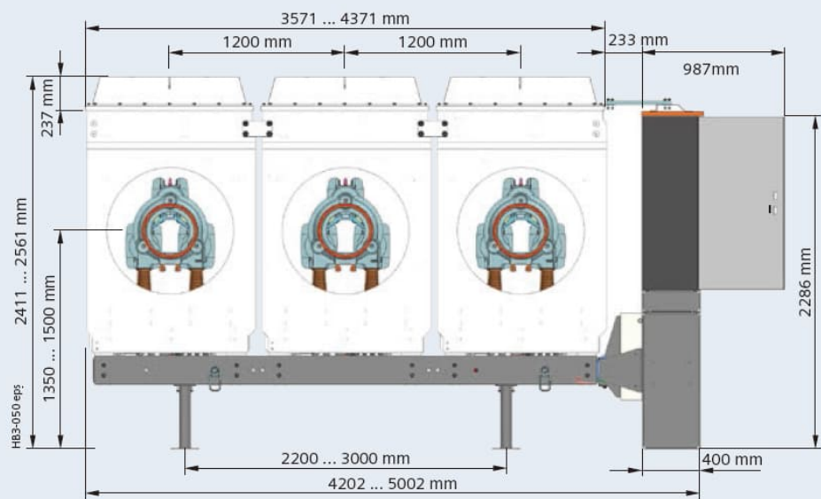
图 8 正视图 标准相间中心距 1200 mm, 可扩展至 1600 mm
