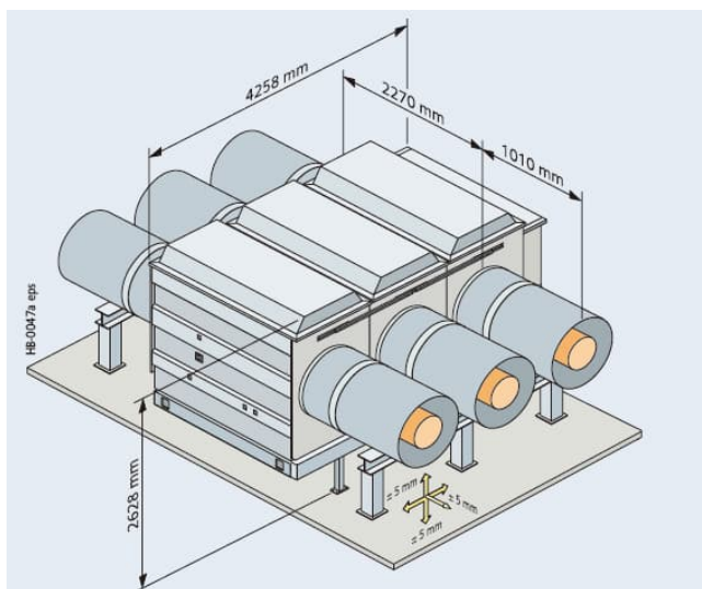
图 31 连接 IPB 的 HB3 型开关设备的典型视图
