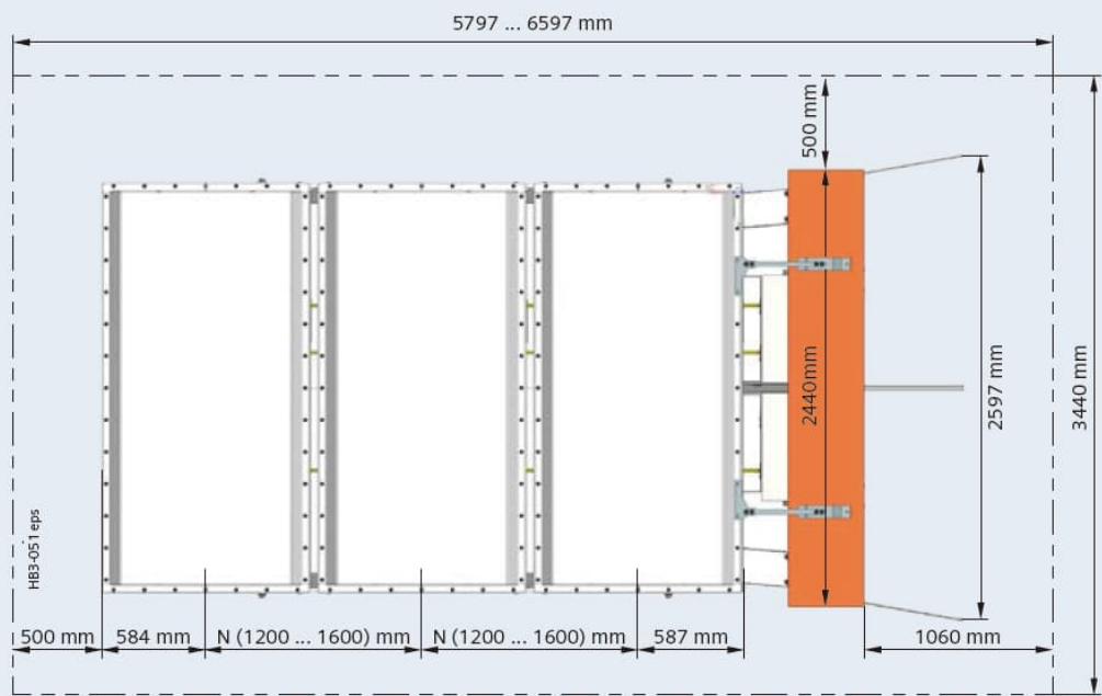
图 9 俯视图，操作控制面板和 前、后及侧面尺寸
