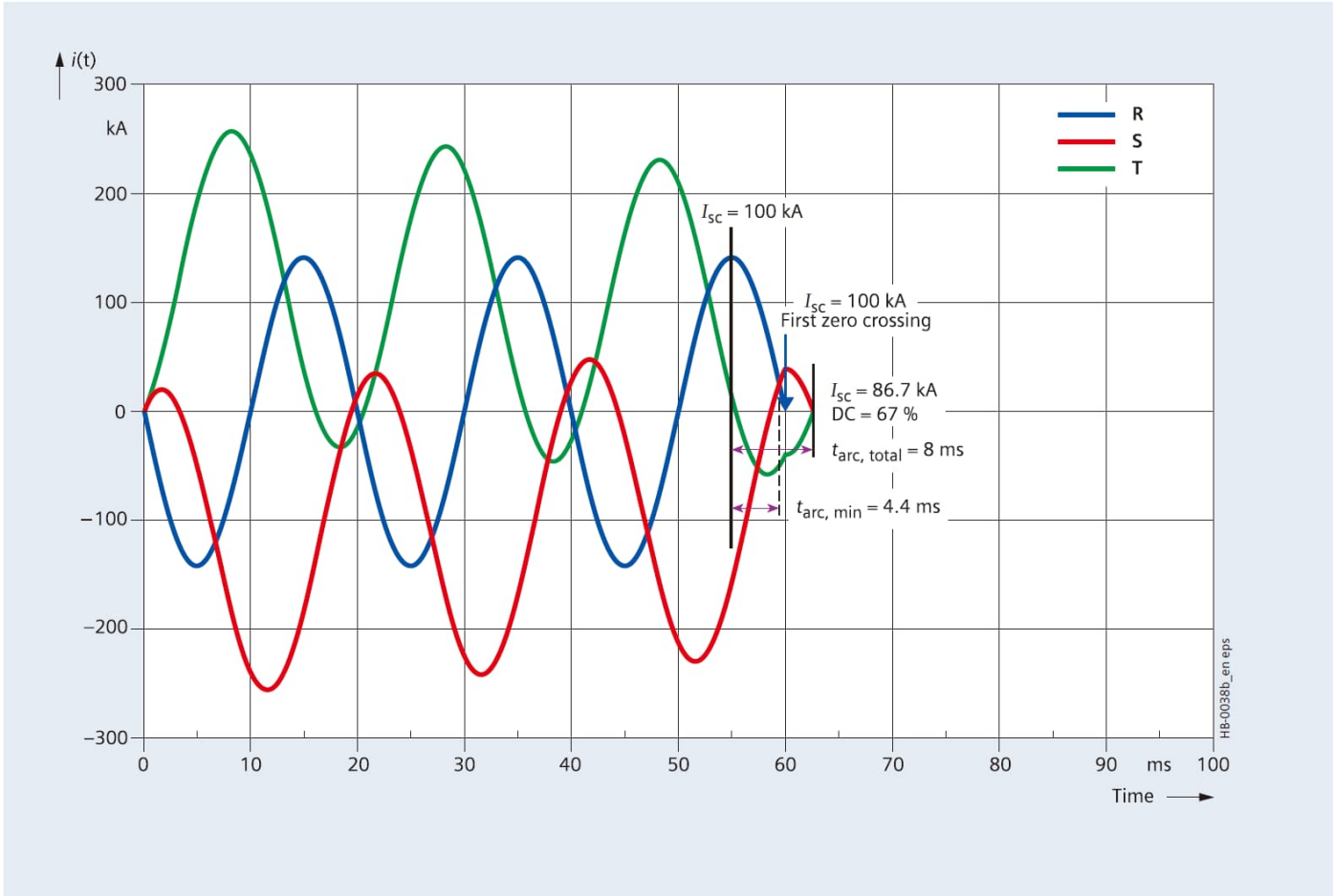
图 54 确认开断能力的短路模拟示例
