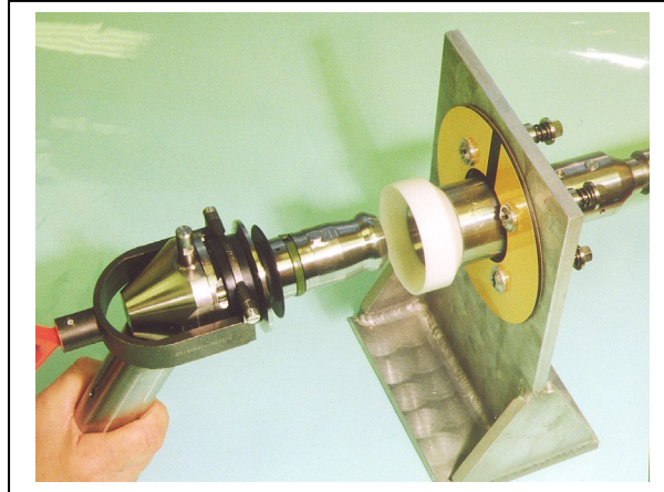
Figure 3: Mini CE ROV Connector
