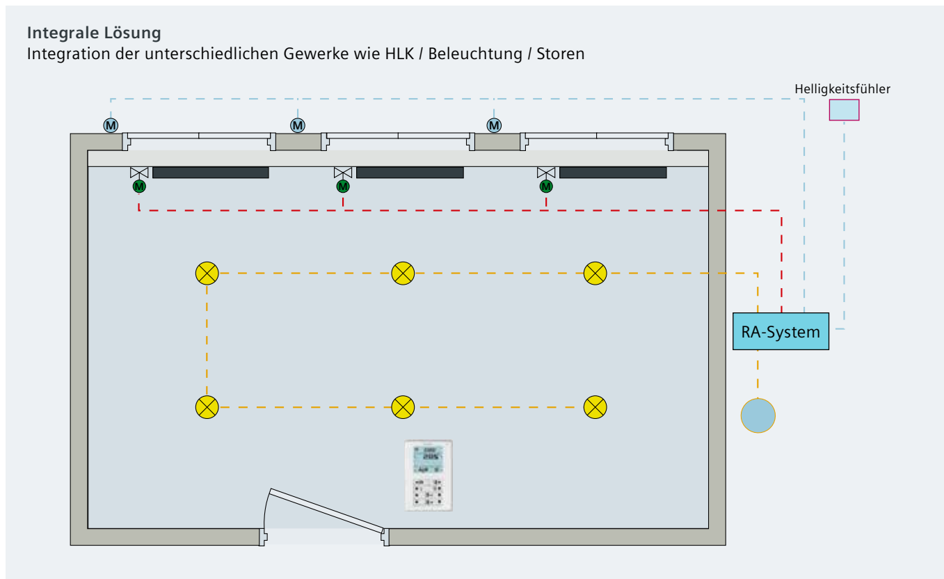
Abb. 3: Gewerkeintegrierte Installation
