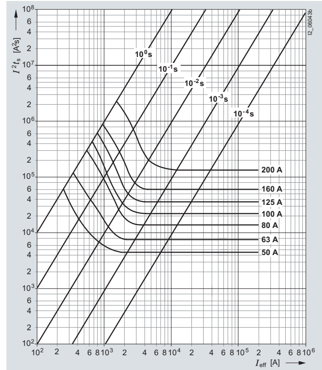
Melting I^2 t_s values diagram
