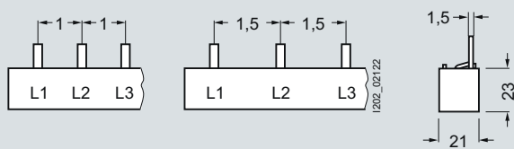
5ST3 710-0HG 5ST3 714-0HG
