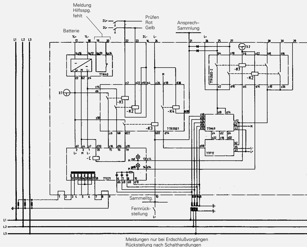
Bild 61 Schaltplan des Erdschlußwischerrelais 7SN70, Ausführung mit 7TM49 und 7TF12 (alte Ausführung)
