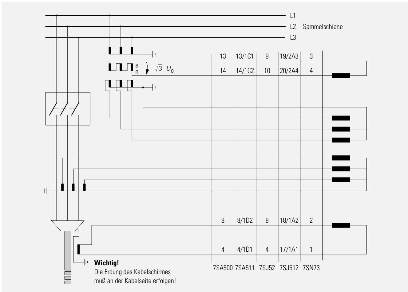
Bild 67 Wandleranschluß wattmetrischer Relais
