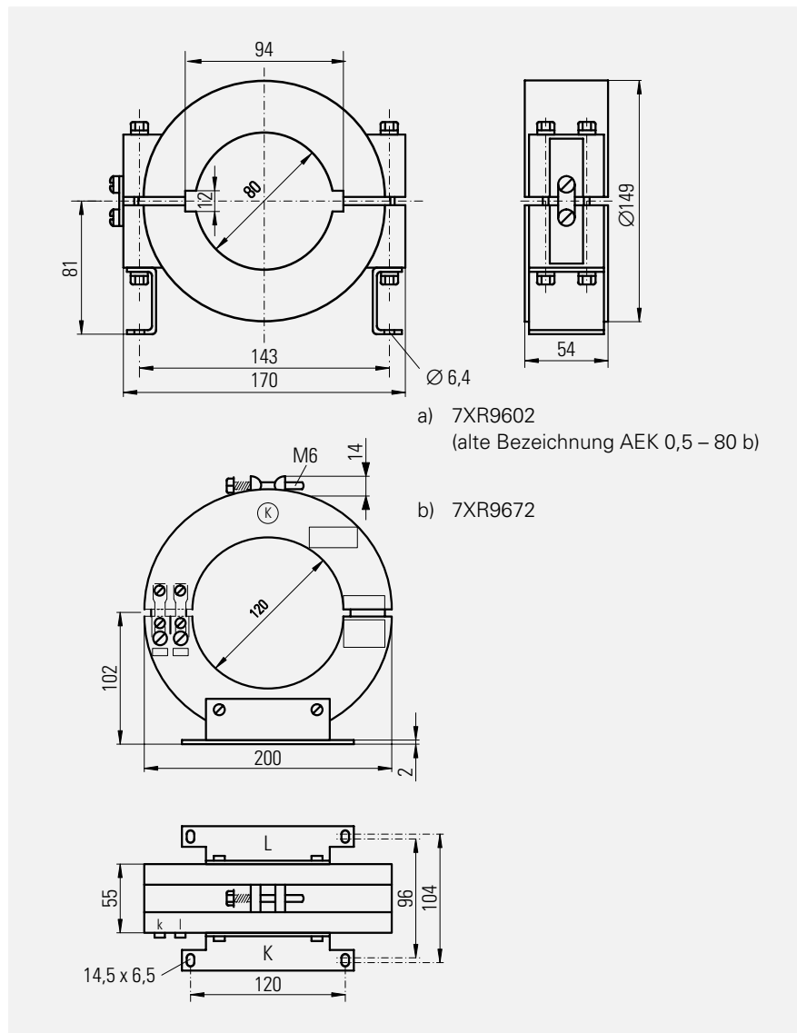
Bild 31 Kabelumbauwandler 7XR96
