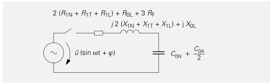
Bild 20 Ersatzschaltung zur Bestimmung der Entladeschwingung der gesunden Phase
