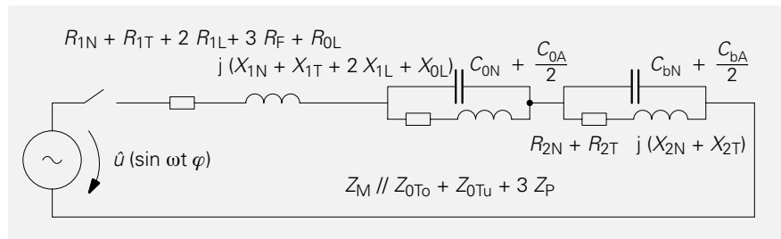
Bild 21 Ersatzschaltung in symmetrischen Komponenten
