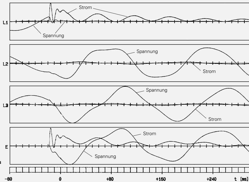
Bild 23 Größen bei gleichen Netzverhältnissen und einem Fehlereintrittszeitpunkt bei einem Winkel von 30 Grad nach dem Spannungsnulldurchgang.
