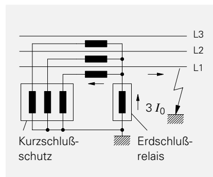
Bild 28 Holmgreenschaltung
