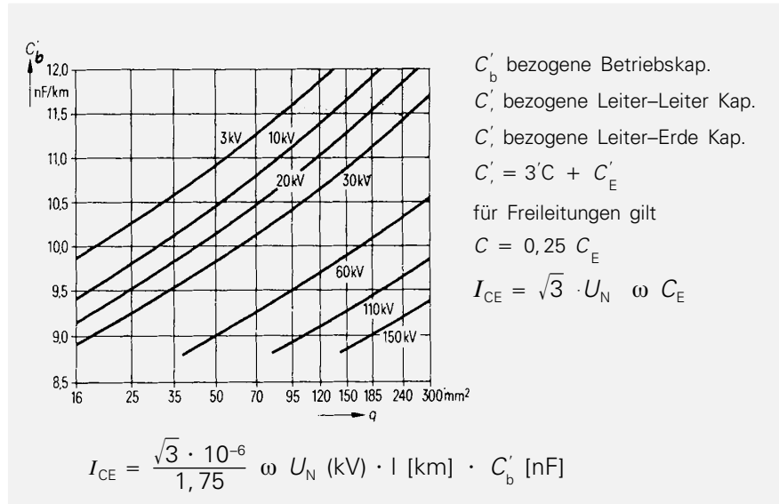
Bild 63 Betriebskapazität C'_b in nF/km je Leiter für Betriebsspannungen bis 150 kV
