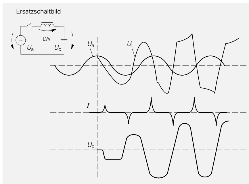
Bild 5 Kippschwingungen
