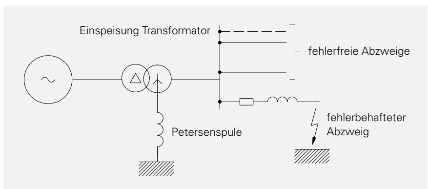
Bild 17 Stichnetz mit Erdschluß, Ersatzschaltbilder
