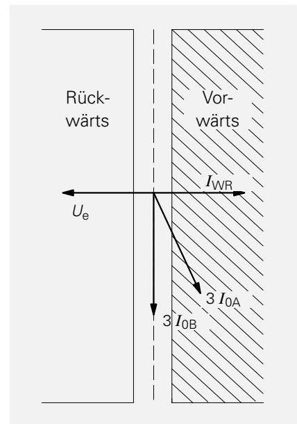
Bild 44 Wirkkomponente des Erdstromes
