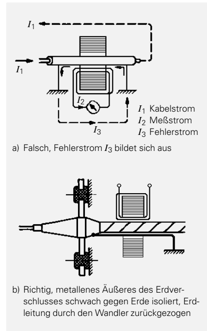
Bild 35 Verlegung der Kabelerdleitung
