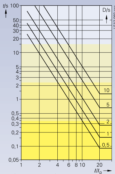
→ Bild 18 I squared T (quadratisch abhängig)
