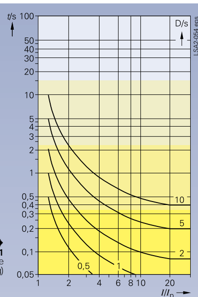
→ Bild 11 Short inverse (kurz abhängig)
