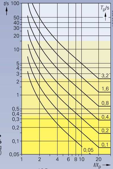
→ Bild 6 Stark abhängig (very inverse)
