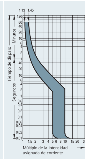
Fig 12.4 - Curva C Protección de conductores, en instalaciones donde se produzcan corrientes de arranque elevadas, por ejemplo: motores, lámparas, etc.
