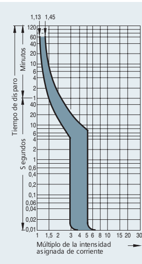
Fig 12.3 - Curva B Protección de gran longitud pero que no permite la inserción de corrientes elevadas de corta duración.
