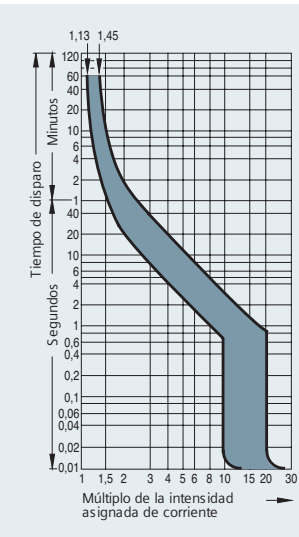
Fig 12.5 - Curva D Protección de conductores, en instalaciones donde se produzcan fuerzas corrientes de impulso, por ejemplo: transformadores, capacitores, etc.
