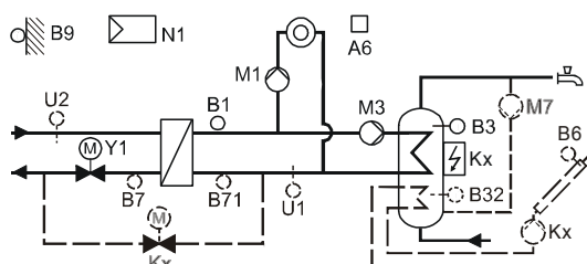
Typ zařízení 4 – pouze RVD145
