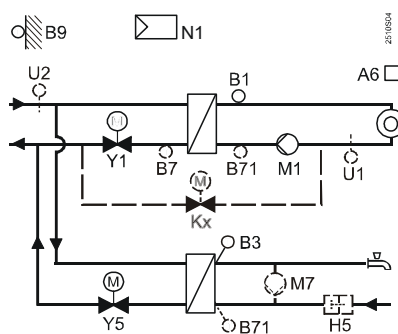
Typ zařízení 6 – pouze RVD145
