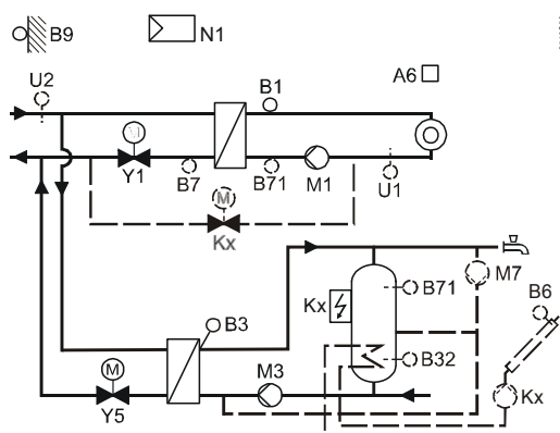
Typ zařízení 8 – pouze RVD145
