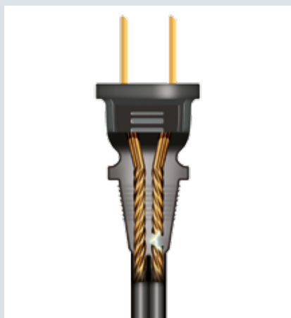
Unterbrechung eines Leiters
