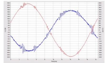
Abbildung 1: Messung (rot) und Berechnung (blau) der Spannung an der Mittelspannungsschiene
