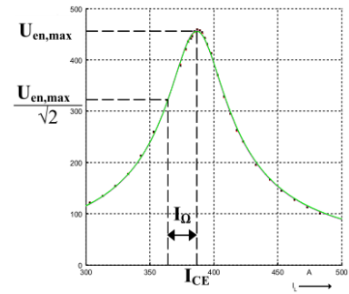
Abbildung 3: Resonanzkurvenauswertung
